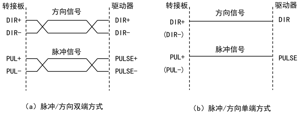
图 3-5 脉冲/方向控制输出示意图
