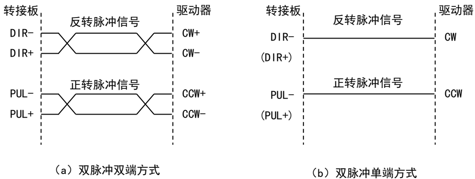
图 3-6 双脉冲控制输出示意图
