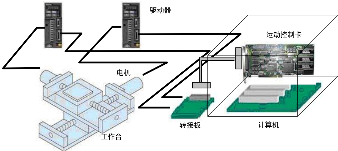
图 1-1 采用 MPC08D 运动控制器组成的控制系统示意图
